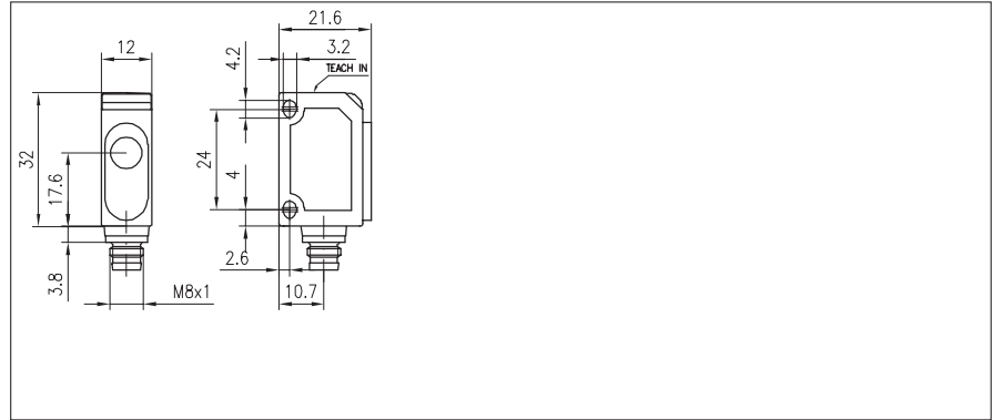
UT 20-I50-PSM 4 UT 20-I50-NSM4
